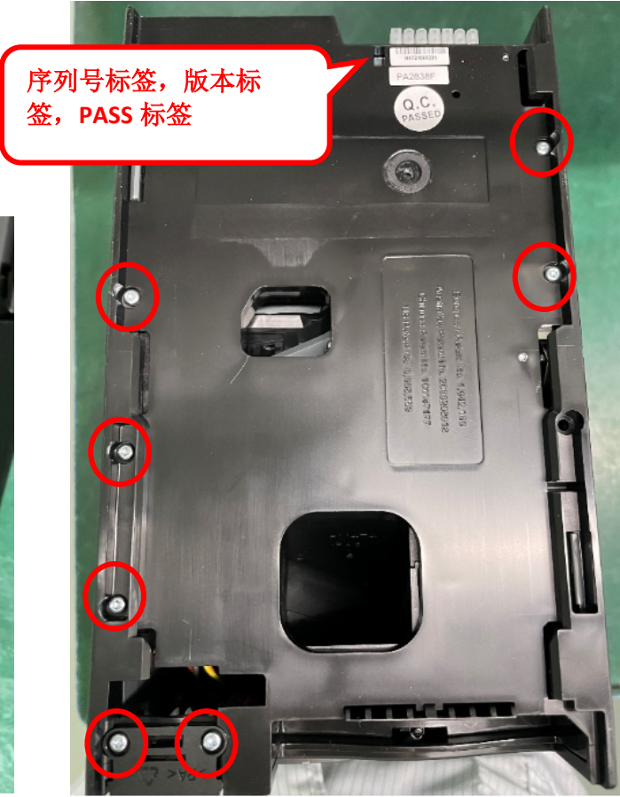
图二，取出铁板组件，检查 3 个标签有无漏贴，信息是否正确，7 颗 SC119 有无漏装
