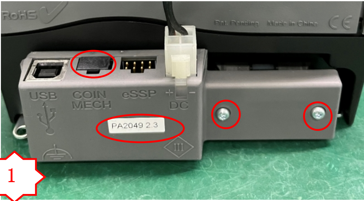
图一，通电 24V 检查单位有无硬币，声音异常，LB2032，2 颗 SC119 有无漏装
